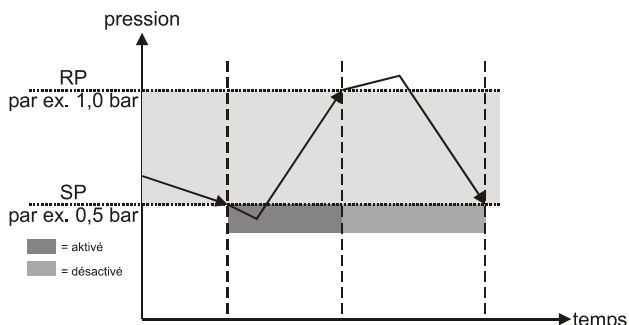
Fig. 60. Contrôleur de pression minimale
