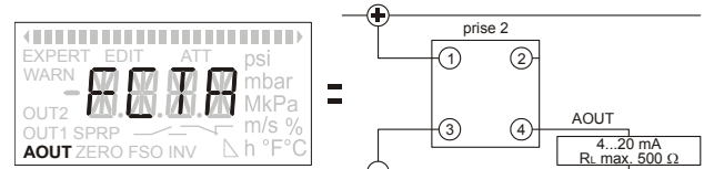
Fig. 15. AOUT sortie analogique 4...20 mA
