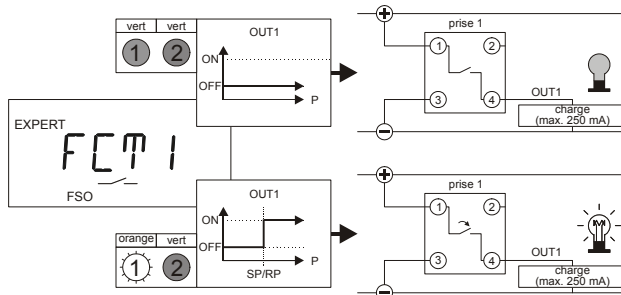
Fig. 7. OUT1 commutateur de tension positive N.O.
