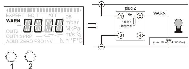
Fig. 17. Sortie WARN (commutateur de tension positive en permanence)
