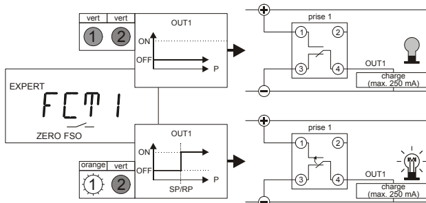
Fig. 9. OUT1 interrupteur push-pull avec charge connectée à 0 V
