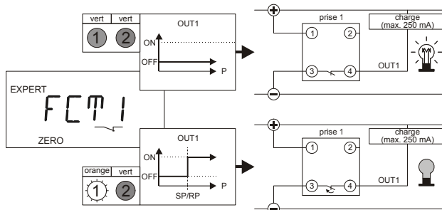
Fig. 6. OUT1 commutateur de 0 V N.F.
