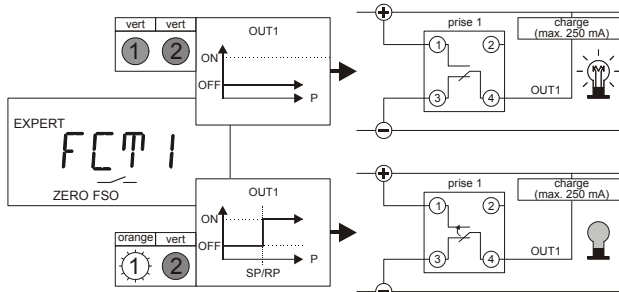
Fig. 11. OUT1 interrupteur push-pull avec charge connectée au secteur
