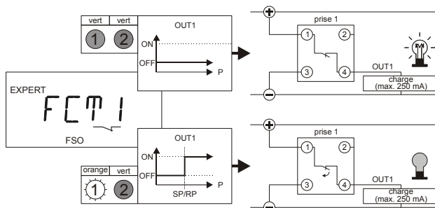
Fig. 8. OUT1 commutateur de tension positive N.F.
