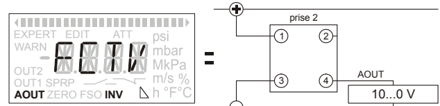
Fig. 14. AOUT sortie analogique 10...0 V
