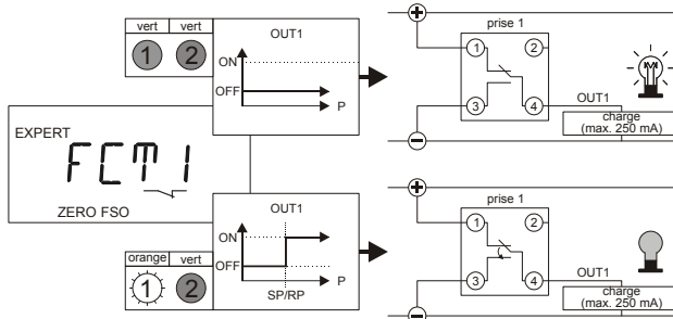
Fig. 10. OUT1 interrupteur push-pull inversé avec charge connectée à 0 V
