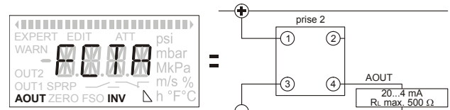
Fig. 16. AOUT sortie analogique 20...4 mA
