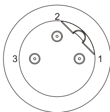
Fig. 4. Prise M12 code B
