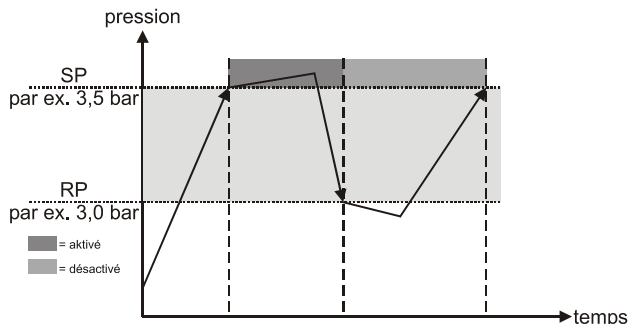
Fig. 58. Contrôleur de pression maximale
