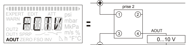
Fig. 13. AOUT sortie analogique 0...10 V
