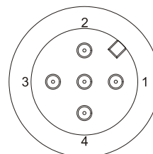
Fig. 3. Prise M12 code A
