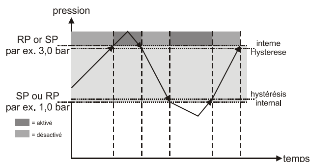
Fig. 62. Fenêtre de contrôle de pression WIN
