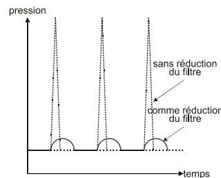
Fig. 20. Effet de réduction du filtre
