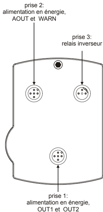
Fig. 1. Modèles PST...-R, vue arrière de la boîte
