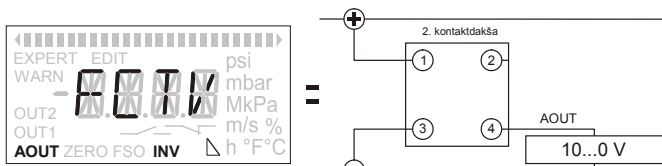
Att. 15. AOUT kā 10...0 V analogā izvade
