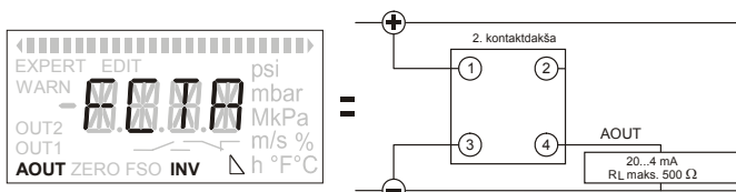
Att. 17. AOUT kā 20...4 mA analogā izvade
