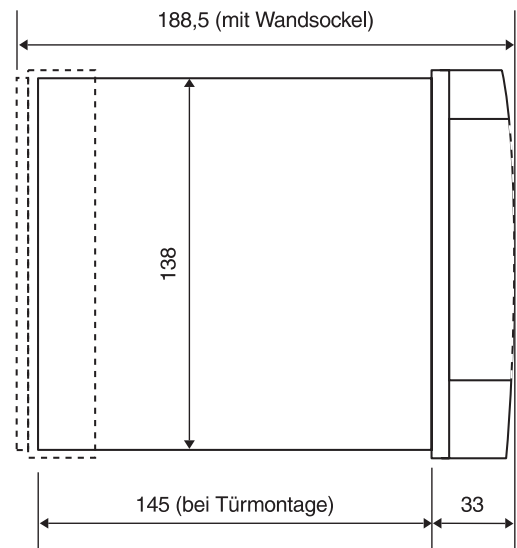
separater Wandsockel (mit Bediengerät)
