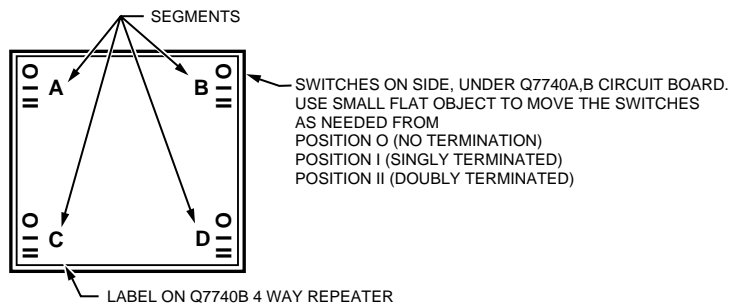
(D) E-Bus Termination network switches in the Q7740A, B Repeaters
